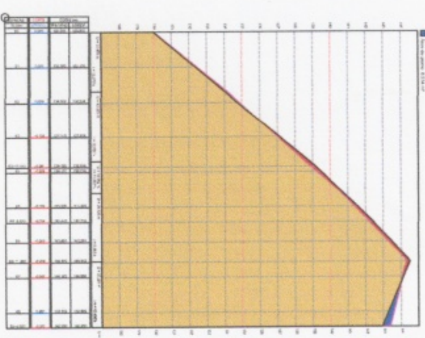
Perfil Longitudinal trecho 02
