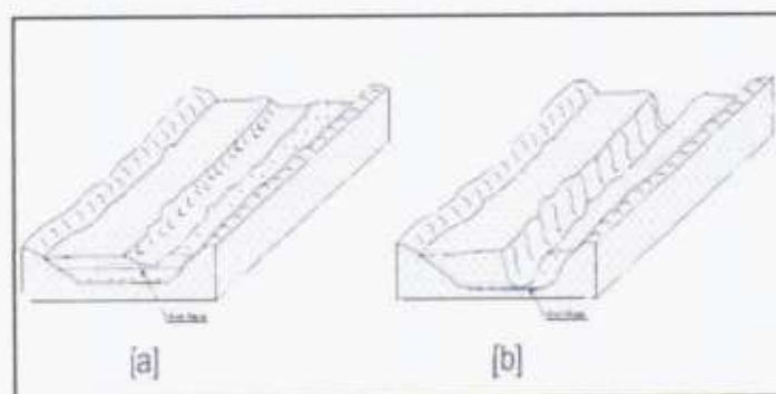
Figura 7- Situação da “calha viva” do riacho em relação aos seus “terraços”: em (a) é favorável ao barramento e em (b) é desfavorável. Fonte: Costa ( 1997)
