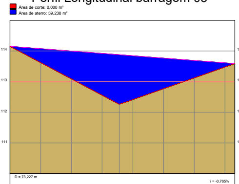
Perfil Longitudinal barragem 05
