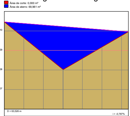
Perfil Longitudinal barragem 04
