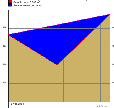
Perfil Longitudinal barragem 03
