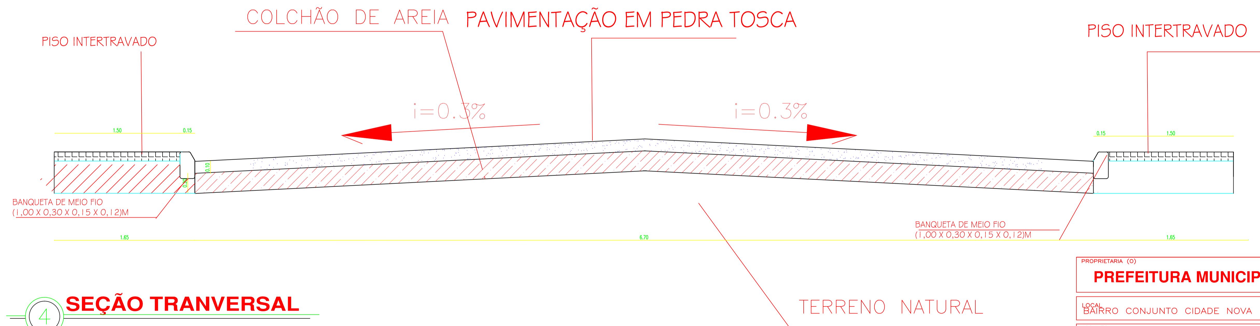
CORTE A/A – TODAS AS RUAS
