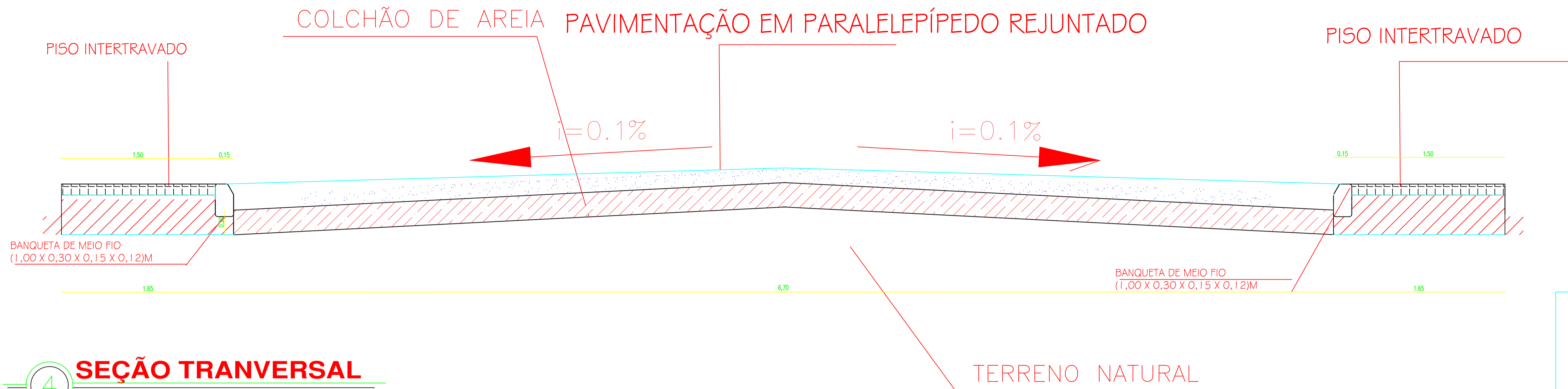
CORTE A/A – TRECHO DA PASSARELA
