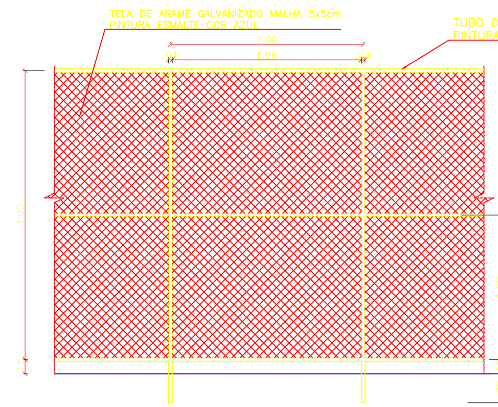
VISTA DO ALAMBRADO (FUNDOS) ESCALA 1:50
