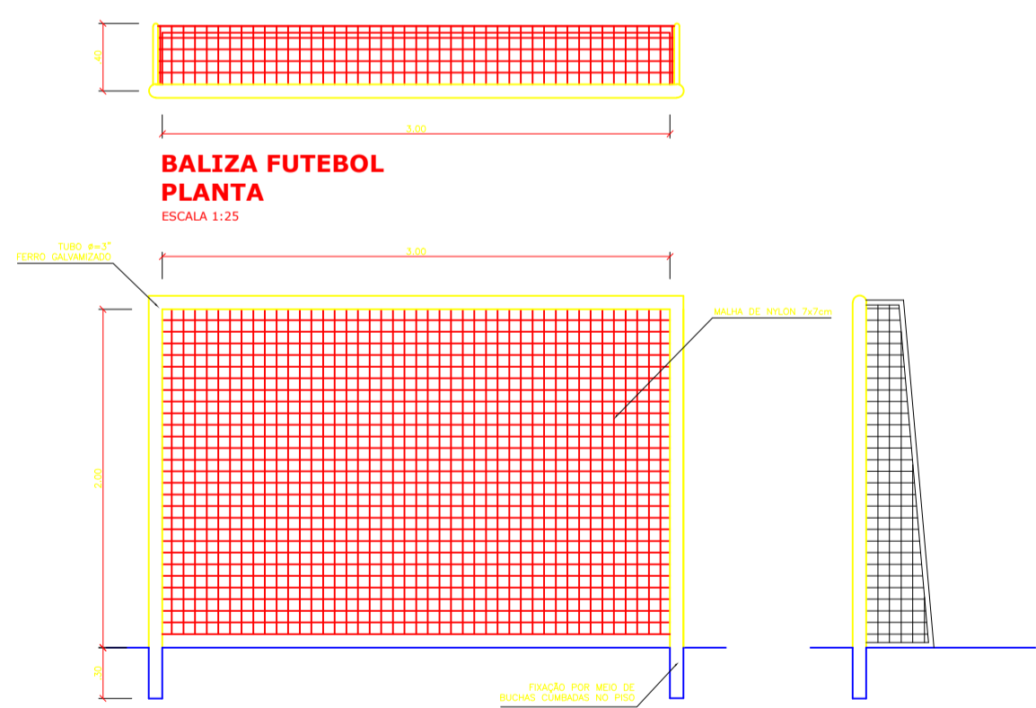
BALIZA FUTEBOL VISTA FRONTAL ESCALA 1:25
