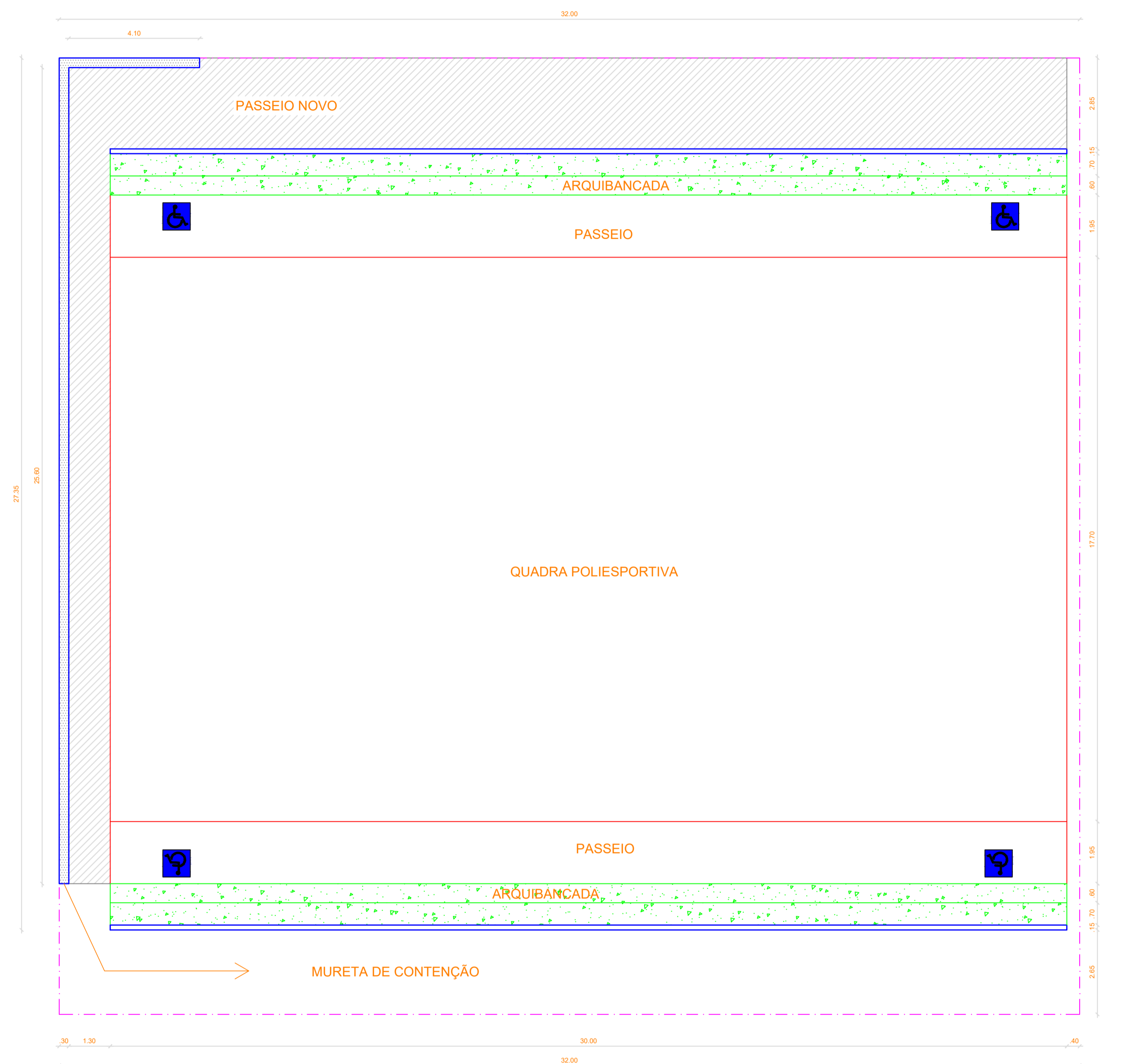
PLANTA BAIXA - CARQUEIJA I ESQ. 1/100
