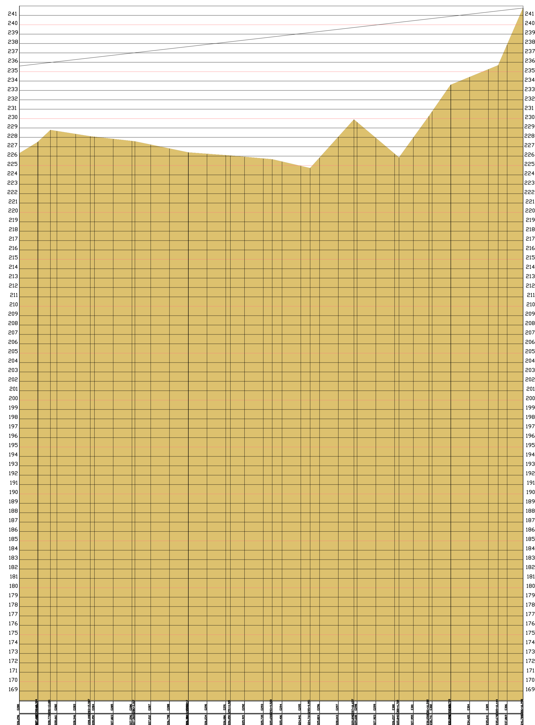
08 PERFIL LONGITUDINAL ESC 1/2000
