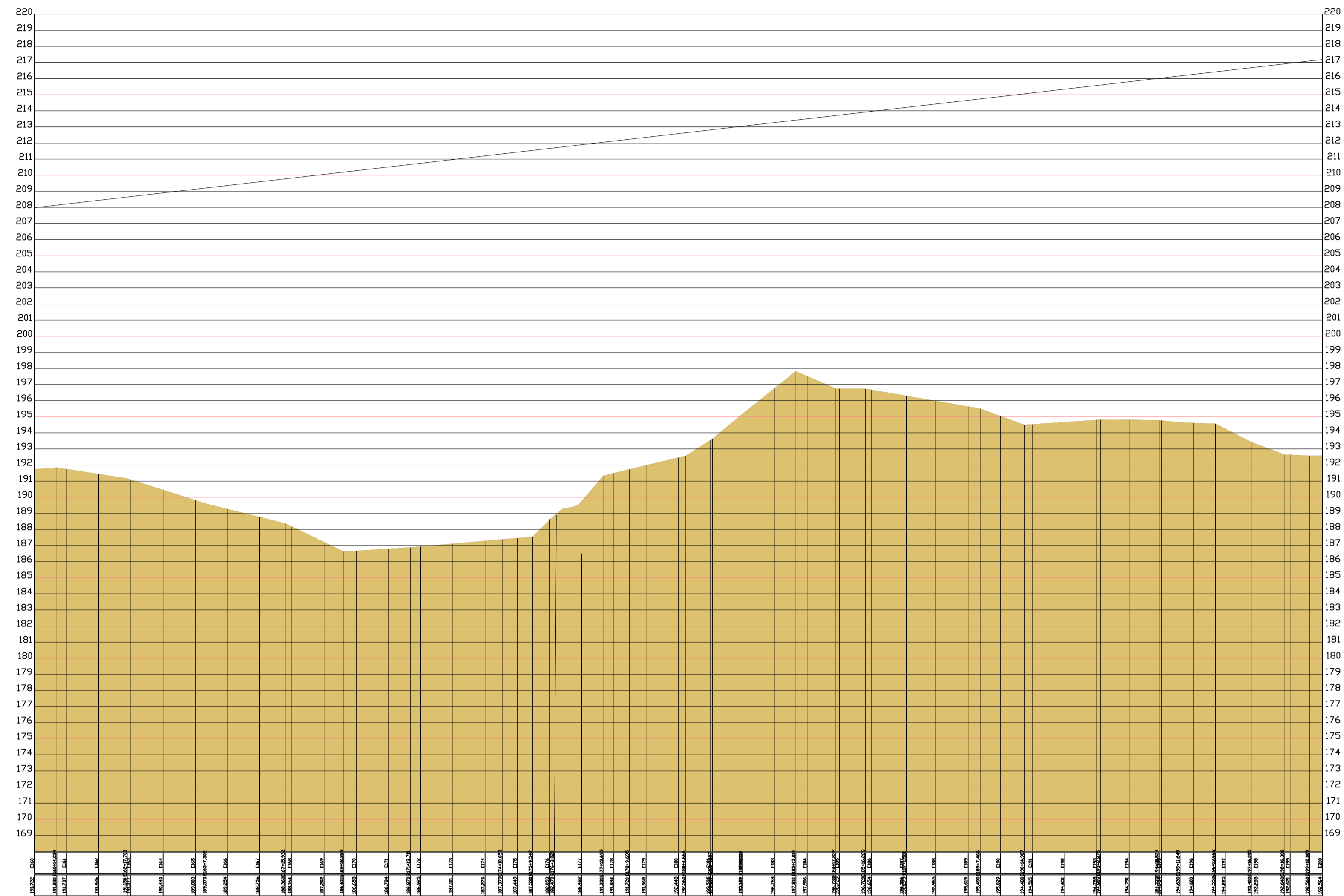
05 PERFIL LONGITUDINAL ESC 1/2000
