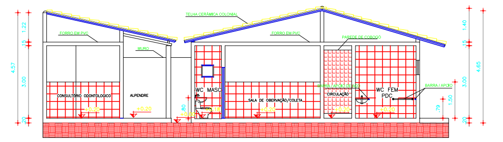
CORTE A-A esc 1/50
