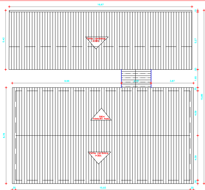
PLANTA BAIXA DE COBERTA A DOMOLIR esc 1/100
