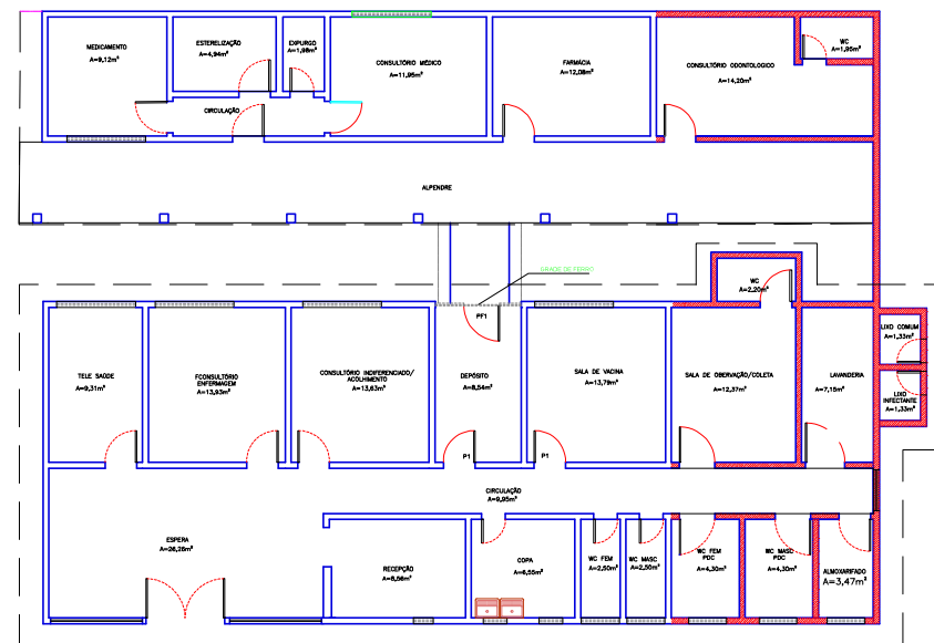
PLANTA BAIXA A CONSTRUIR esc 1/100
