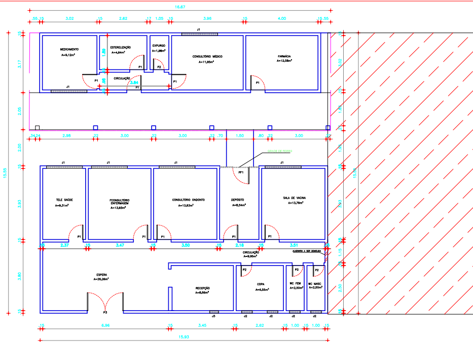
PLANTA BAIXA - A DOMOLIR esc 1/100
