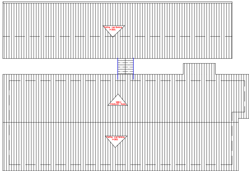
PLANTA BAIXA DE COBERTA A CONSTRUIR esc 1/100
