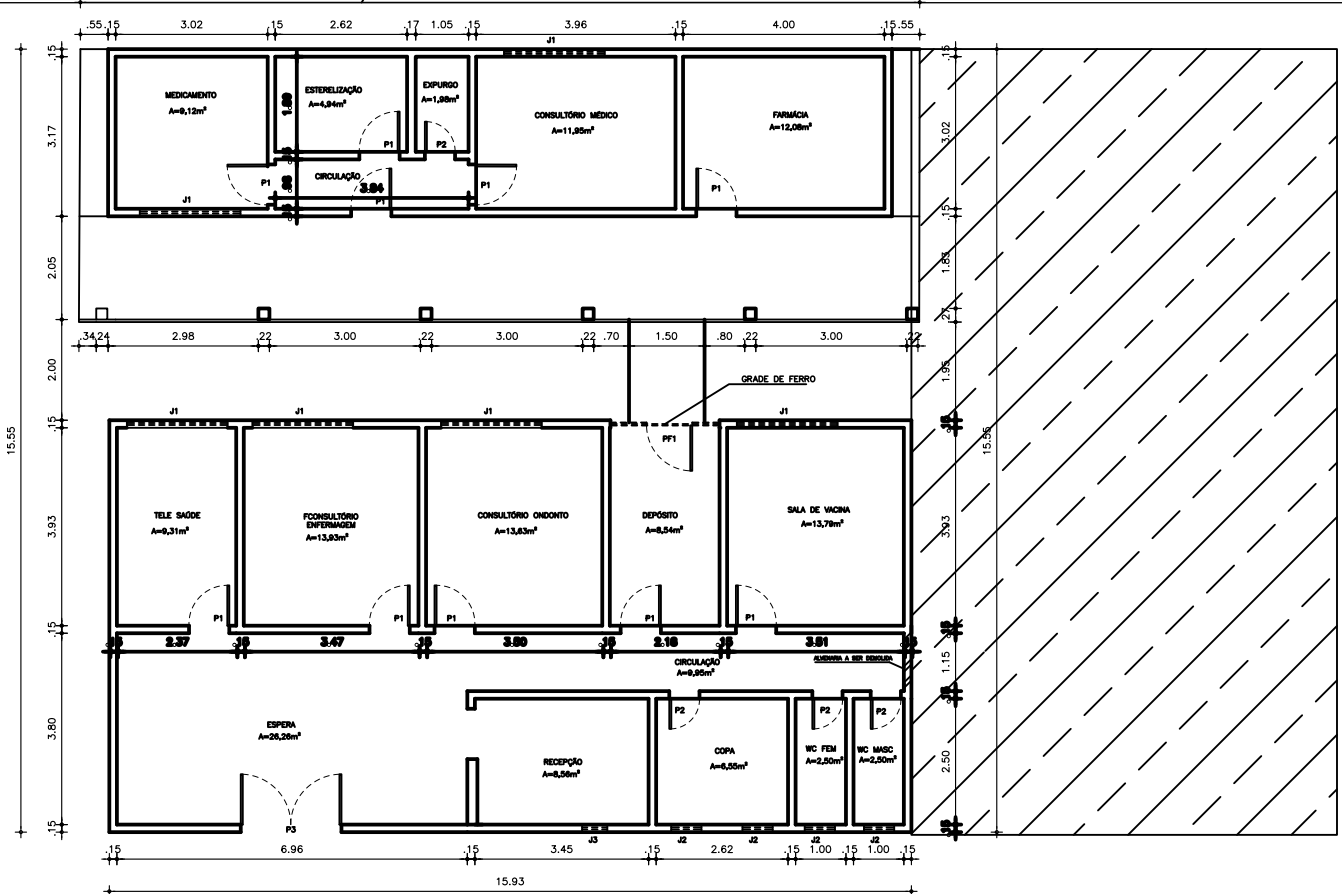
PLANTA BAIXA - A DEMILIR esc 1/175
