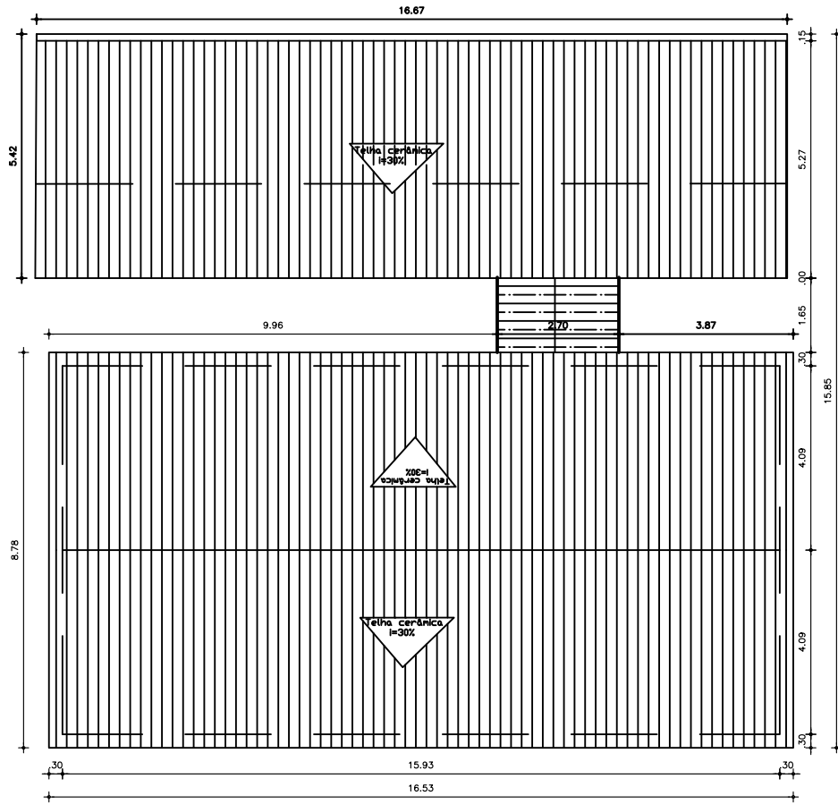
PLANTA BAIXA DE COBERTA A DOMILIR esc 1/150
